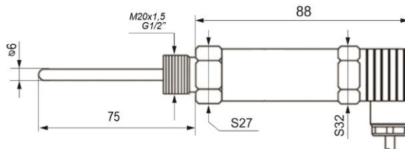
Рисунок 1 – Термопреобразователь с цифровым выходом T.Pt – RS – DIN – 6 – 75 – (-70/+200)
